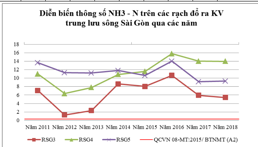
Biểu đồ 11: Diễn biến \text{N-NH}_3 trên các rạch đổ ra khu vực trung lưu sông Sài Gòn qua các năm
