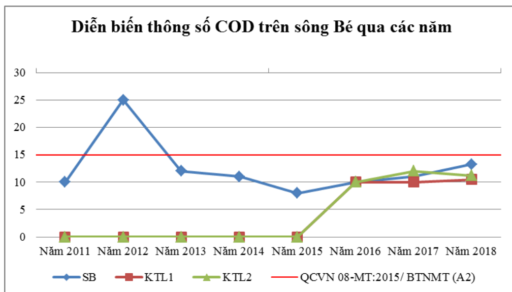
Biểu đồ 40: Diễn biến mức độ ô nhiễm COD trên sông Bé và kênh thủy lợi qua các năm
