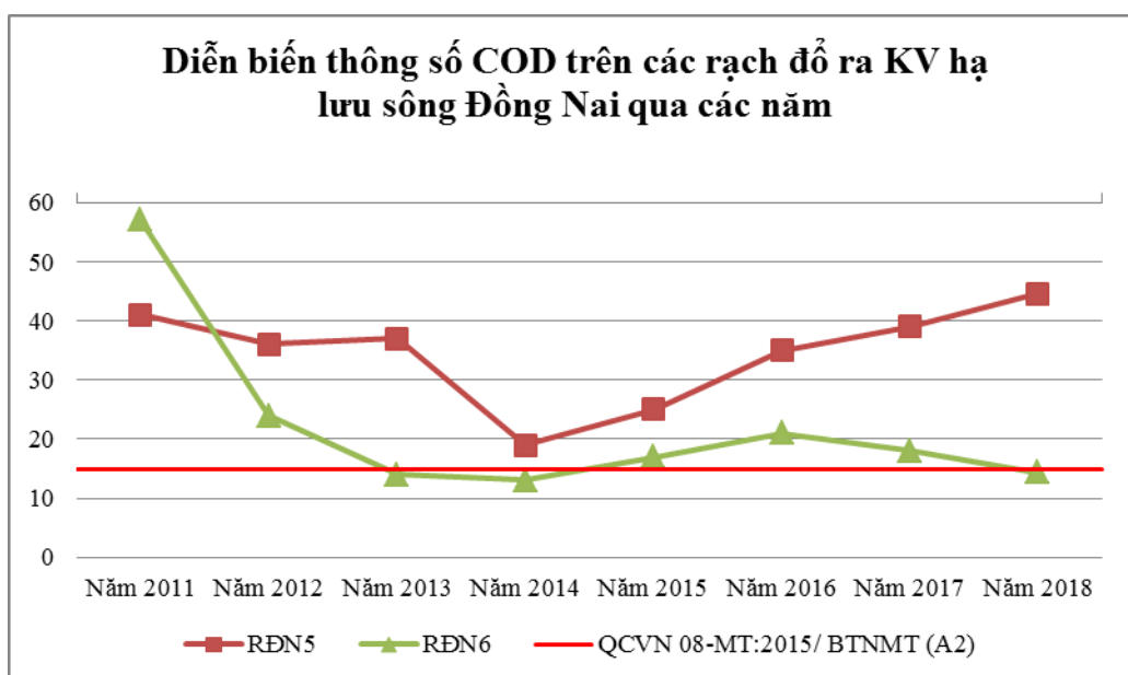
Biểu đồ 32: Diễn biến COD trên các rạch đổ ra khu vực hạ lưu sông Đồng Nai qua các năm
