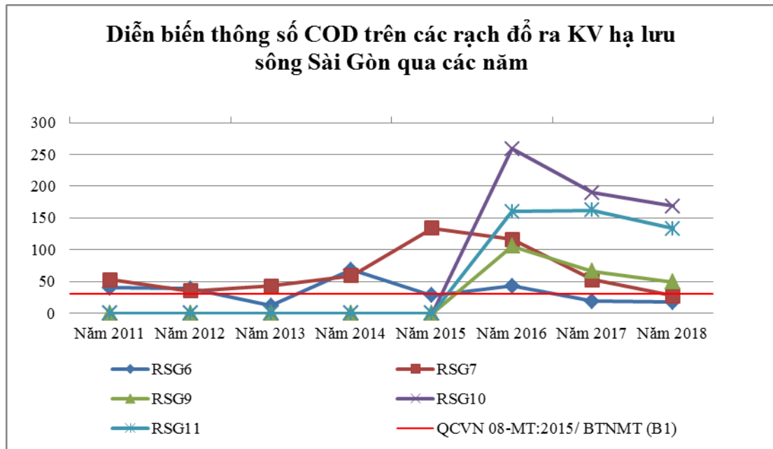
Biểu đồ 16: Diễn biến COD trên các rạch đổ ra khu vực hạ lưu sông Sài Gòn qua các năm
