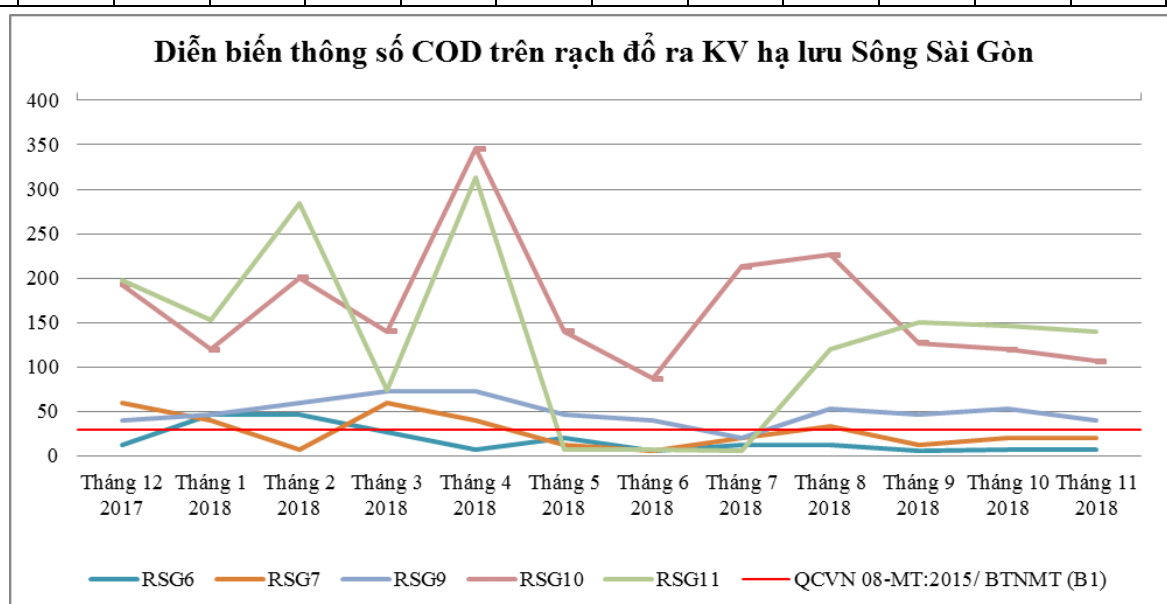
Biểu đồ 14: Diễn biến COD trên các rạch đổ ra khu vực hạ lưu sông Sài Gòn năm 2018
