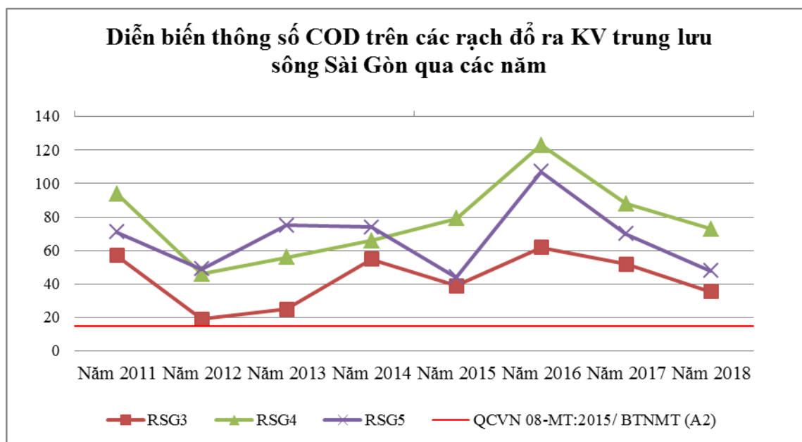
Biểu đồ 12: Diễn biến COD trên các rạch đổ ra khu vực trung lưu sông Sài Gòn qua các năm
