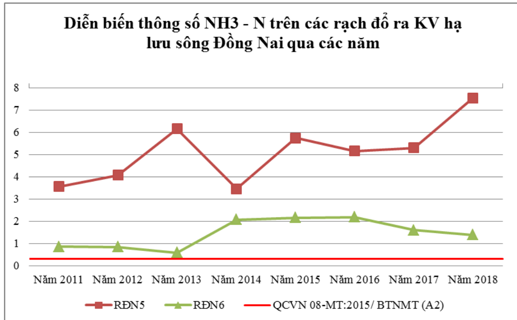
Biểu đồ 31: Diễn biến N-NH 3 trên các rạch đổ ra khu vực hạ lưu sông Đồng Nai qua các năm
