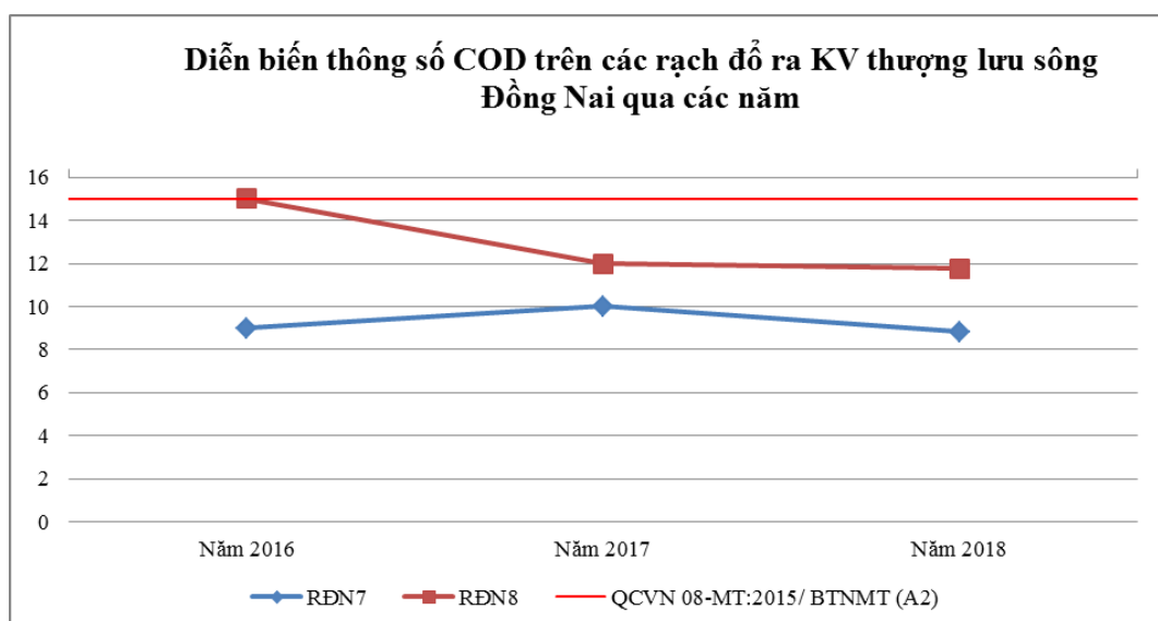
Biểu đồ 24: Diễn biến COD trên các rạch đổ ra khu vực thượng lưu sông Đồng Nai qua các năm
