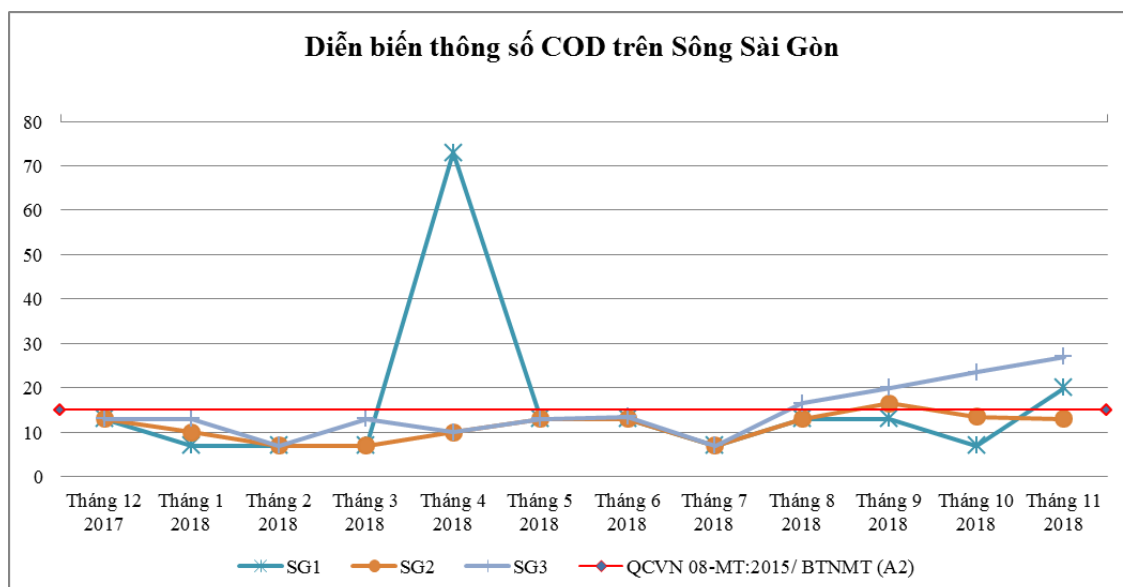
Biểu đồ 2: Diễn biến mức độ ô nhiễm COD trên các đoạn sông Sài Gòn năm 2018
