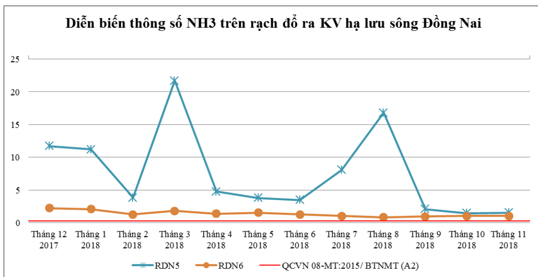
Biểu đồ 29: Diễn biến N-NH 3 trên các rạch đổ ra khu vực hạ lưu sông Đồng Nai năm 2018
