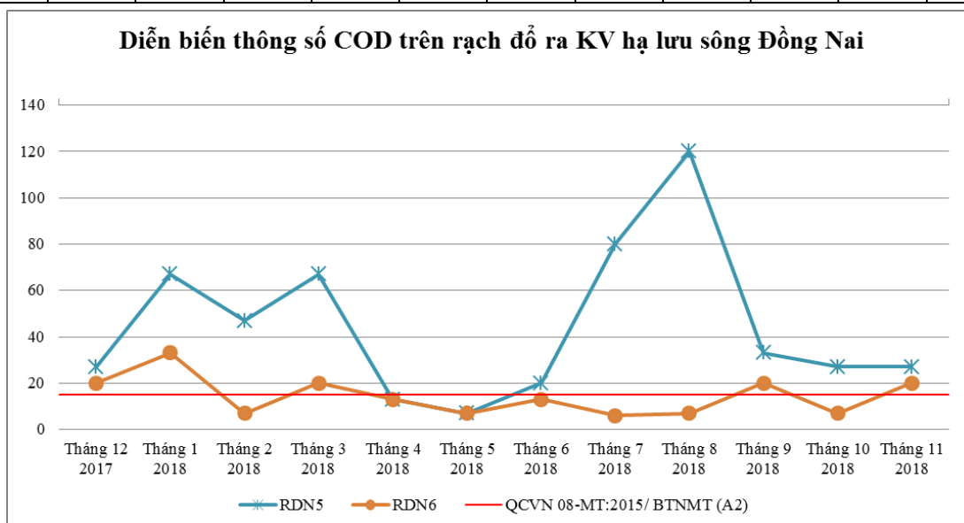
Biểu đồ 30: Diễn biến COD trên các rạch đổ ra khu vực hạ lưu sông Đồng Nai năm 2018
