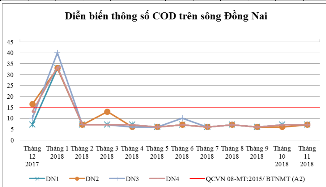
Biểu đồ 18: Diễn biến COD trên các đoạn sông Đồng Nai năm 2018
