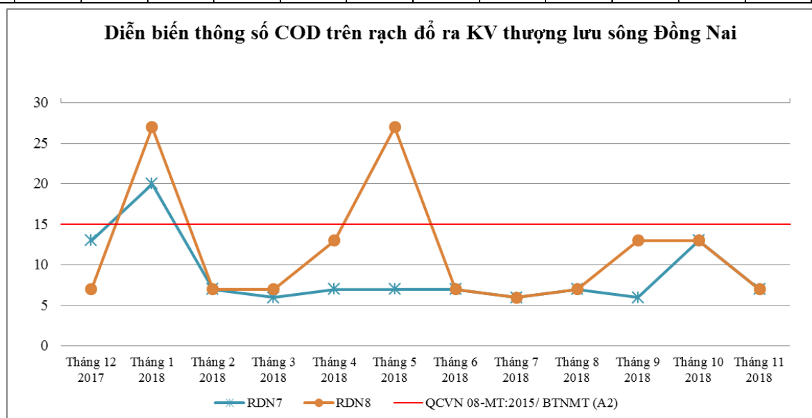
Biểu đồ 22: Diễn biến COD trên các rạch đổ ra khu vực thượng lưu sông Đồng Nai năm 2018
