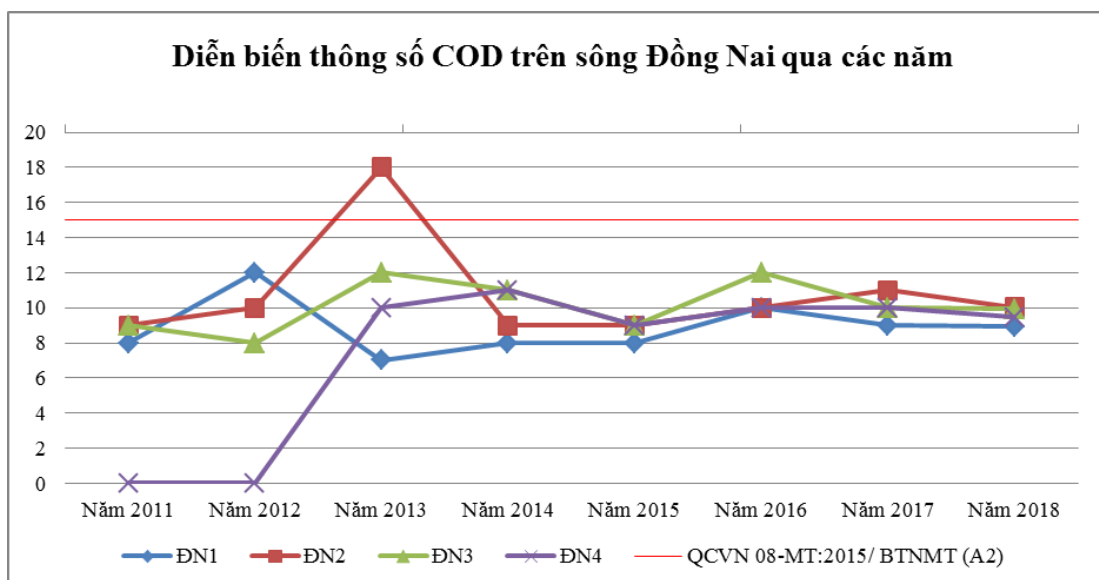
Biểu đồ 20: Diễn biến COD trên các đoạn sông Đồng Nai qua các năm
