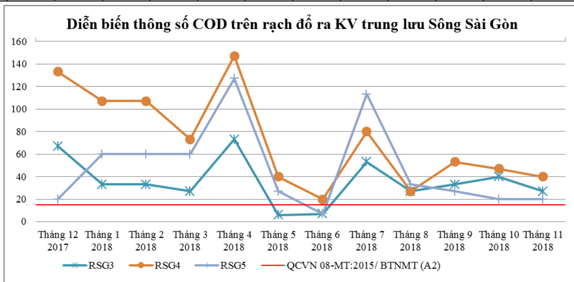
Biểu đồ 10: Diễn biến COD trên các rạch đổ ra khu vực trung lưu sông Sài Gòn năm 2018
