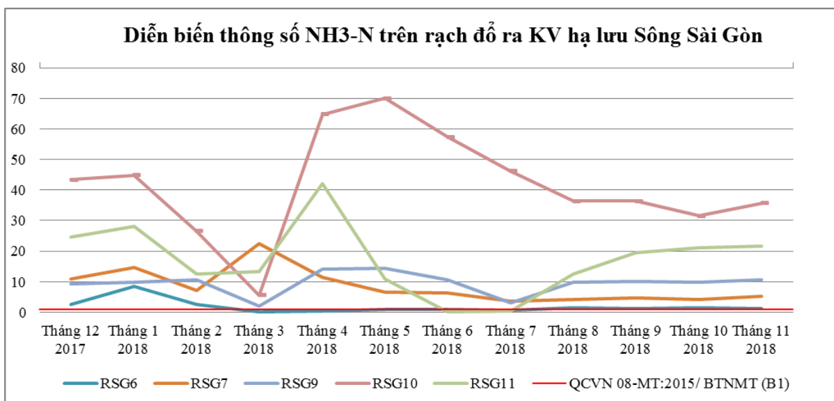
Biểu đồ 13: Diễn biến N-NH 3 trên các rạch đổ ra khu vực hạ lưu sông Sài Gòn năm 2018
