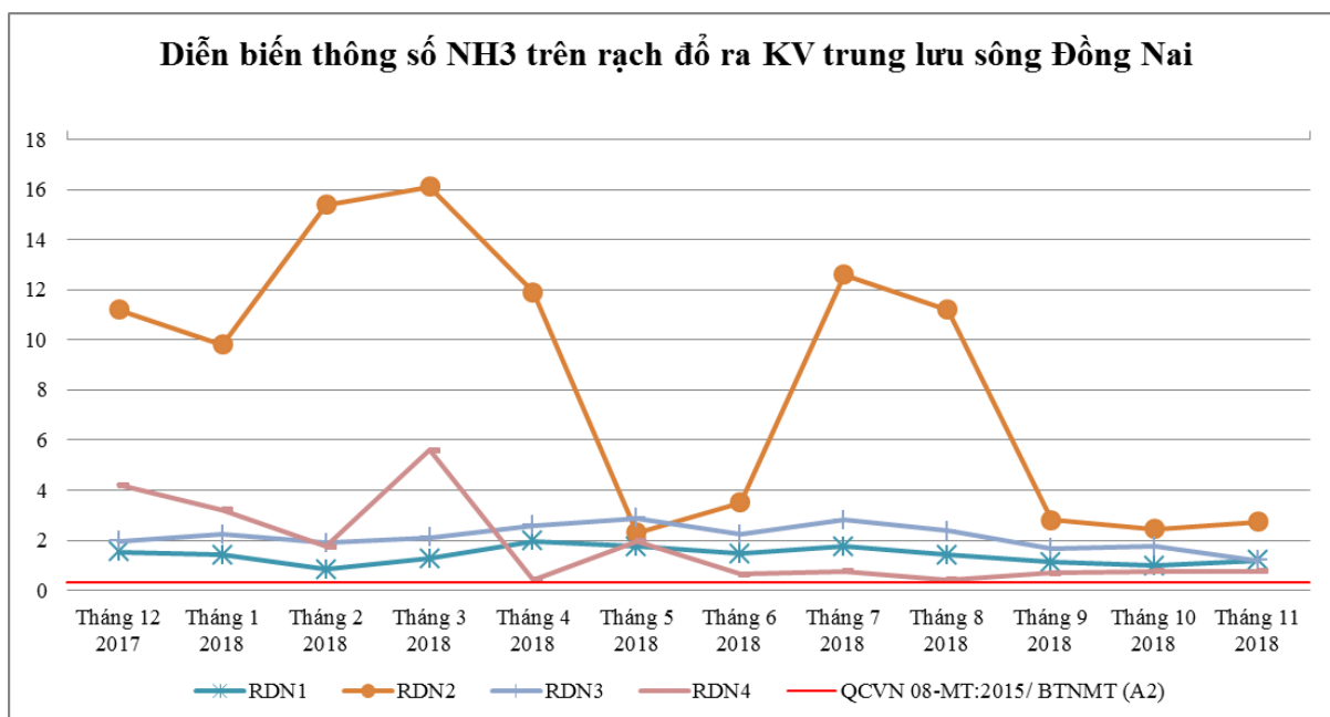
Biểu đồ 25: Diễn biến N-NH 3 trên các rạch đổ ra khu vực trung lưu sông Đồng Nai năm 2018
