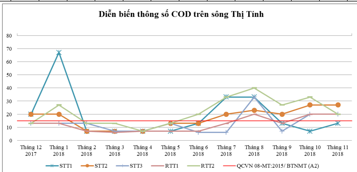
Biểu đồ 34: Diễn biến mức độ ô nhiễm COD trên sông Thị Tính năm 2018
