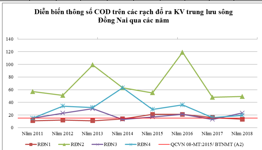
Biểu đồ 28: Diễn biến COD trên các rạch đổ ra khu vực trung lưu sông Đồng Nai qua các năm
