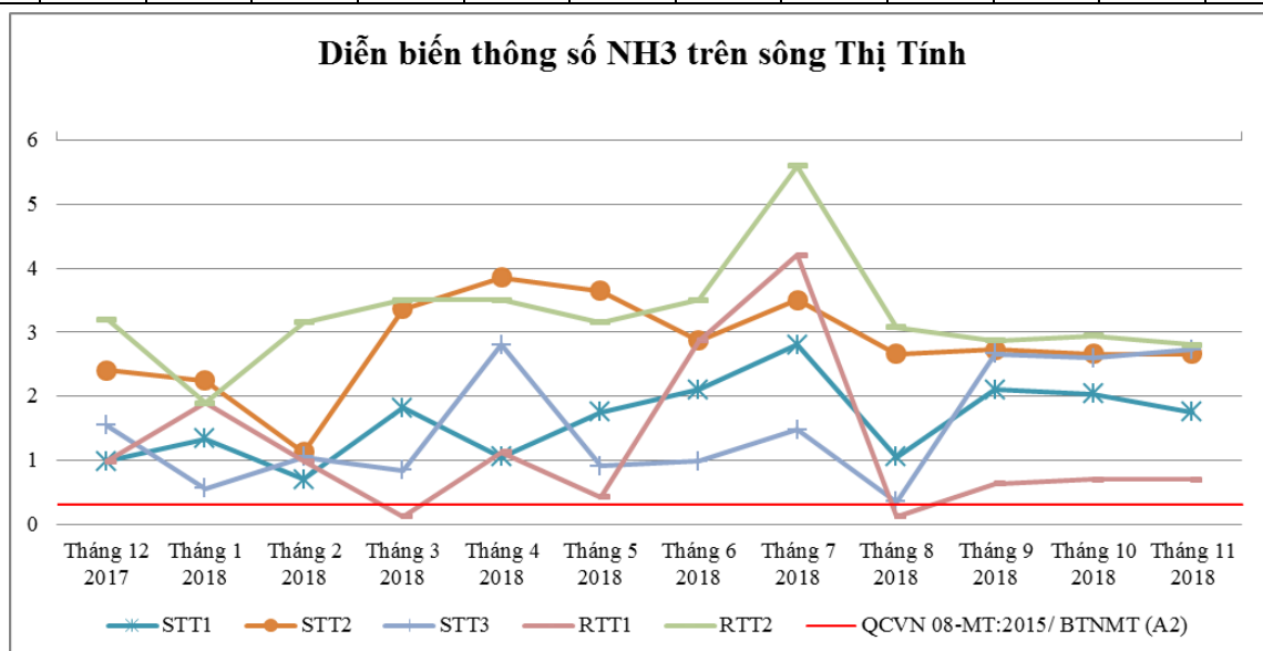
Biểu đồ 33: Diễn biến mức độ ô nhiễm N-NH 3 trên sông Thị Tính năm 2018
