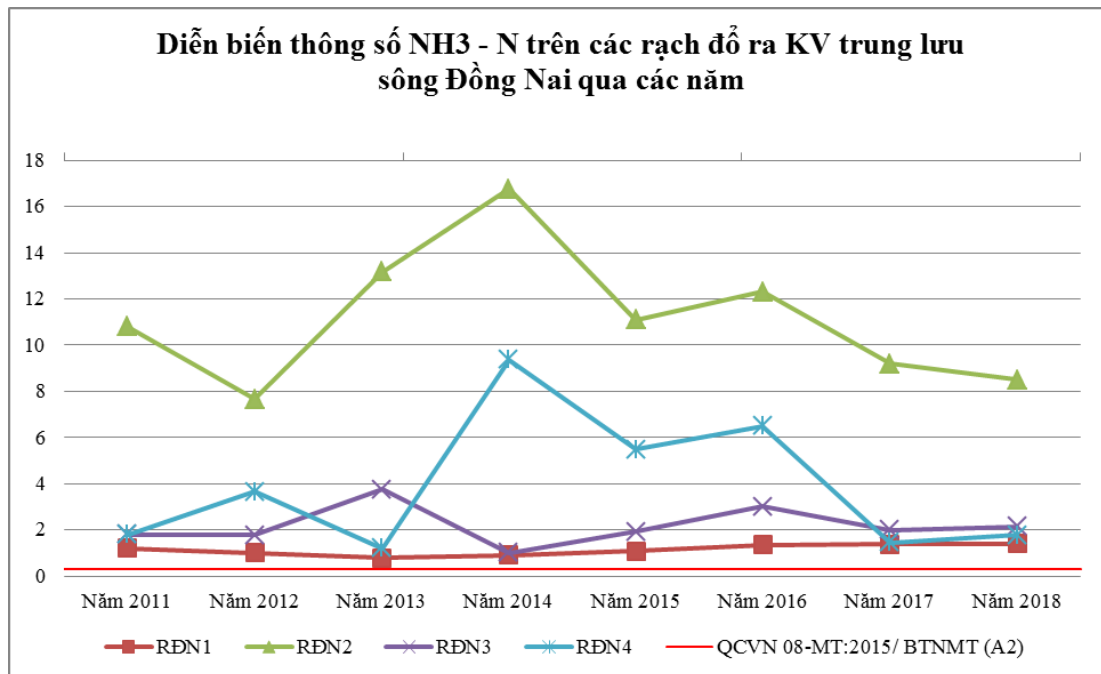
Biểu đồ 27: Diễn biến \text{N-NH}_3 trên các rạch đổ ra khu vực trung lưu sông Đồng Nai qua các năm
