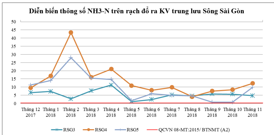
Biểu đồ 9: Diễn biến N-NH 3 trên các rạch đổ ra khu vực trung lưu sông Sài Gòn năm 2018
