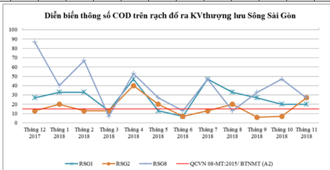
Biểu đồ 6: Diễn biến COD trên các rạch đổ ra khu vực thượng lưu sông Sài Gòn năm 2018
