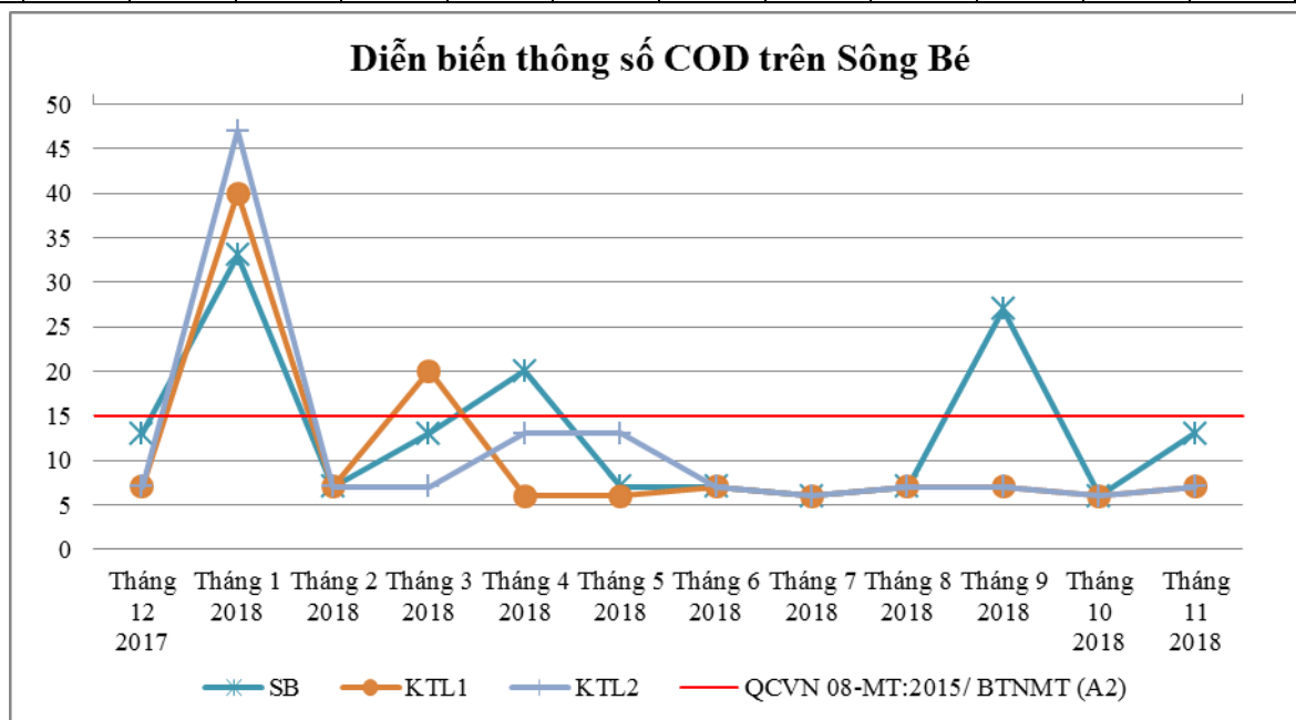
Biểu đồ 38: Diễn biến mức độ ô nhiễm COD trên sông Bé và kênh thủy lợi năm 2018
