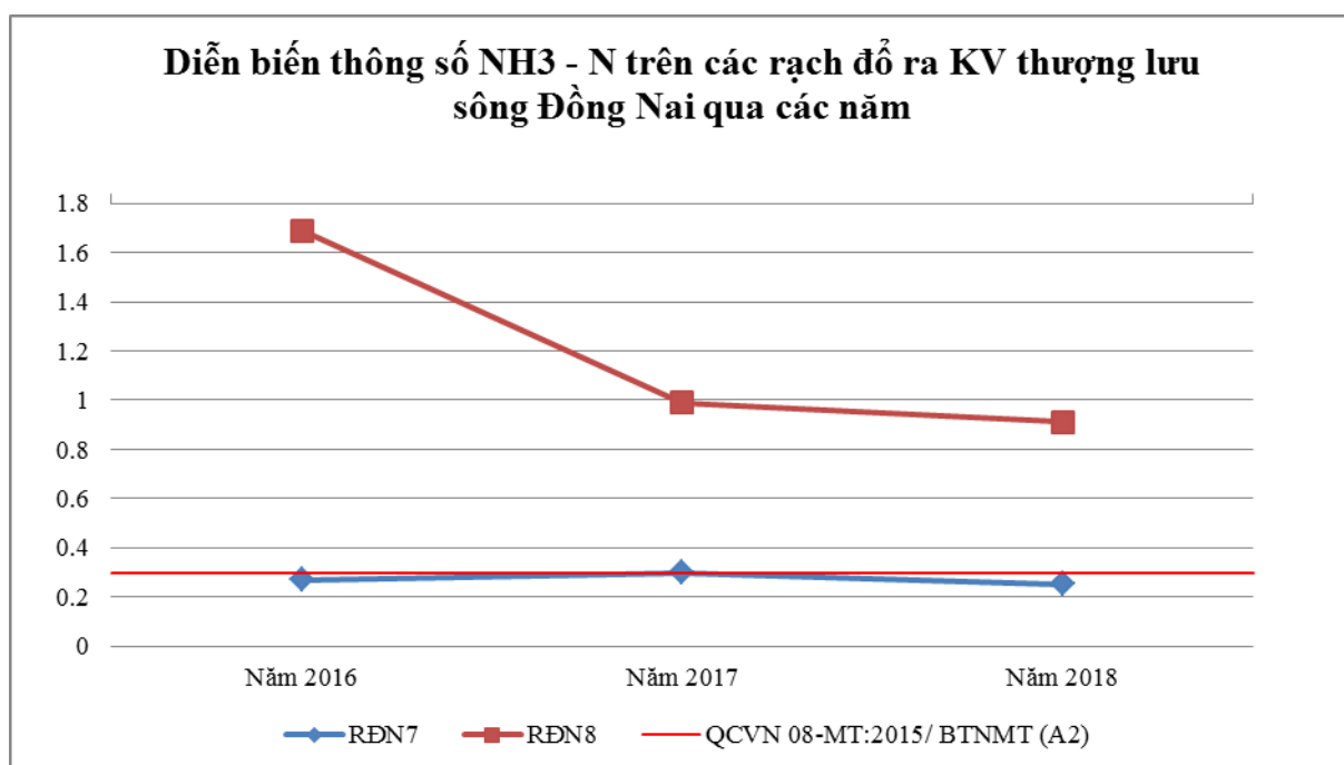
Biểu đồ 23: Diễn biến N-NH 3 trên các rạch đổ ra khu vực thượng lưu sông Đồng Nai qua các năm
