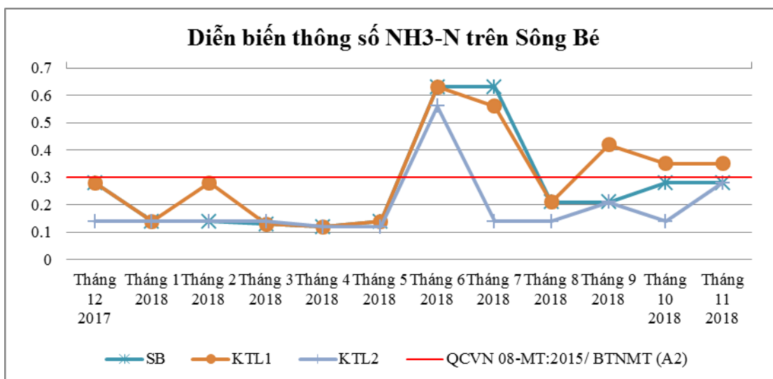
Biểu đồ 37: Diễn biến mức độ ô nhiễm N-NH 3 trên sông Bé và kênh thủy lợi năm 2018
