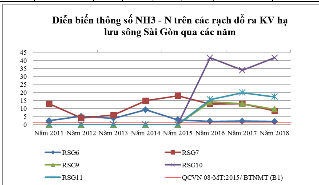
Biểu đồ 15: Diễn biến \text{N-NH}_3 trên các rạch đổ ra khu vực hạ lưu sông Sài Gòn qua các năm
