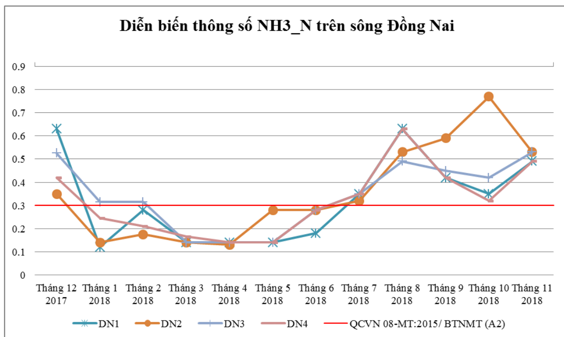
Biểu đồ 17: Diễn biến N-NH 3 trên các đoạn sông Đồng Nai năm 2018
