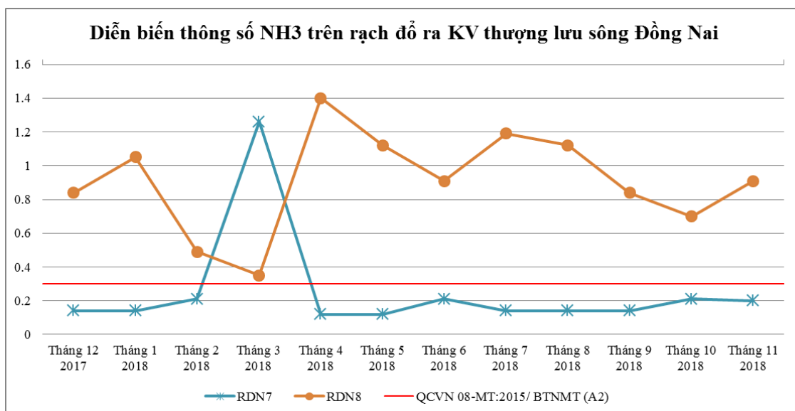
Biểu đồ 21: Diễn biến N-NH 3 trên các rạch đổ ra khu vực thượng lưu sông Đồng Nai năm 2018
