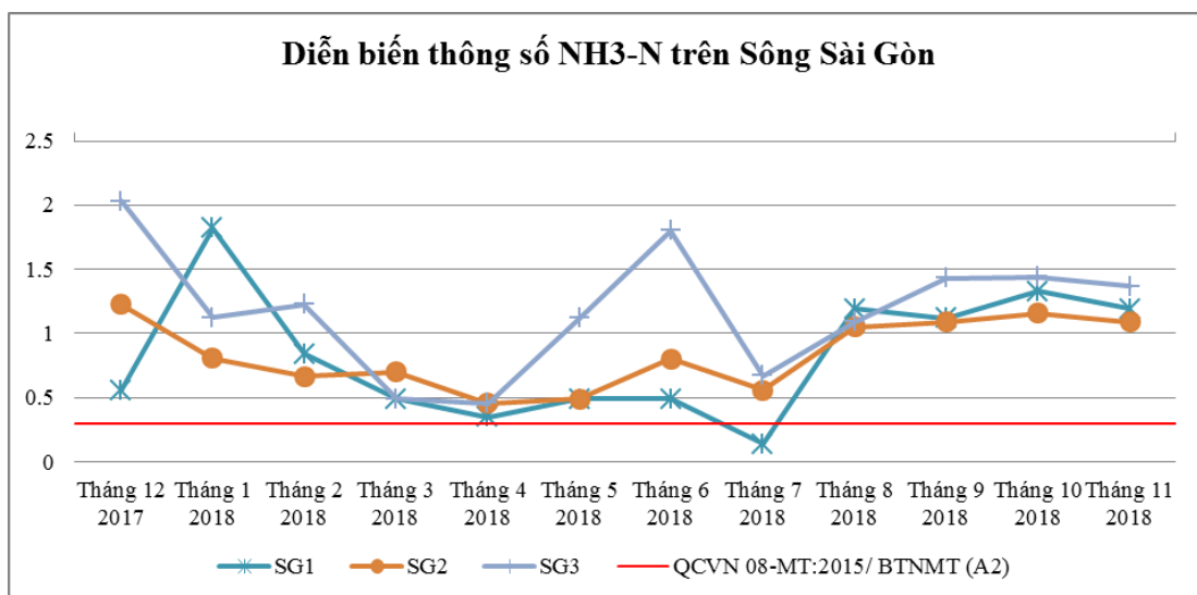
Biểu đồ 1: Diễn biến mức độ ô nhiễm Amoni trên các đoạn sông Sài Gòn năm 2018
