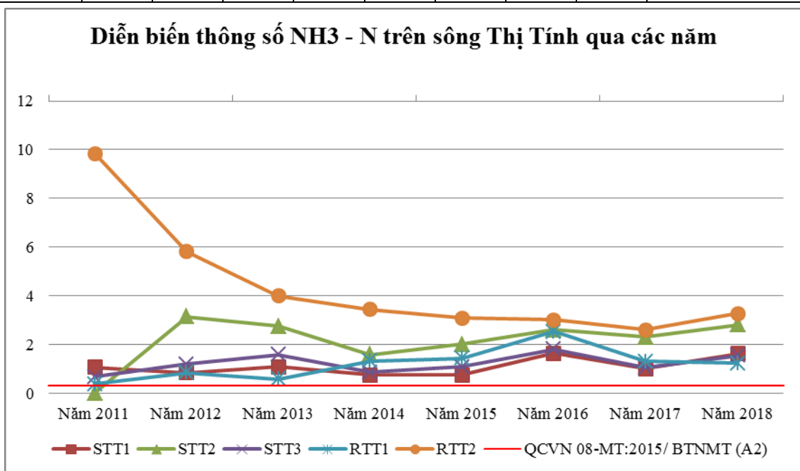
Biểu đồ 35: Diễn biến mức độ ô nhiễm \text{N-NH}_3 trên sông Thị Tính qua các năm
