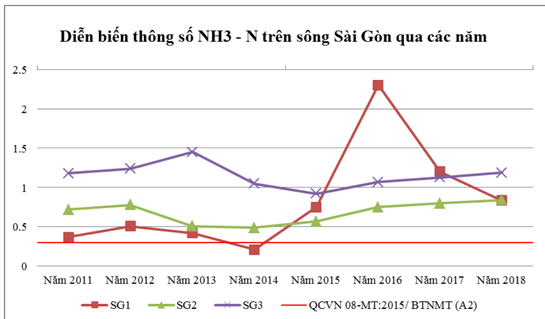
Biểu đồ 3: Diễn biến mức độ ô nhiễm N-NH 3 trên các đoạn sông Sài Gòn qua các năm
