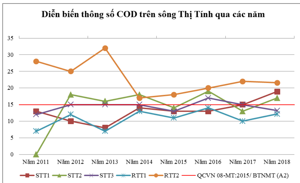
Biểu đồ 36: Diễn biến mức độ ô nhiễm COD trên sông Thị Tính qua các năm
