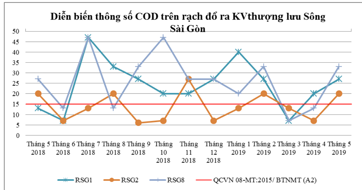
Biểu đồ 4: Diễn biến COD trên các rạch đổ ra khu vực thượng lưu sông Sài Gòn
