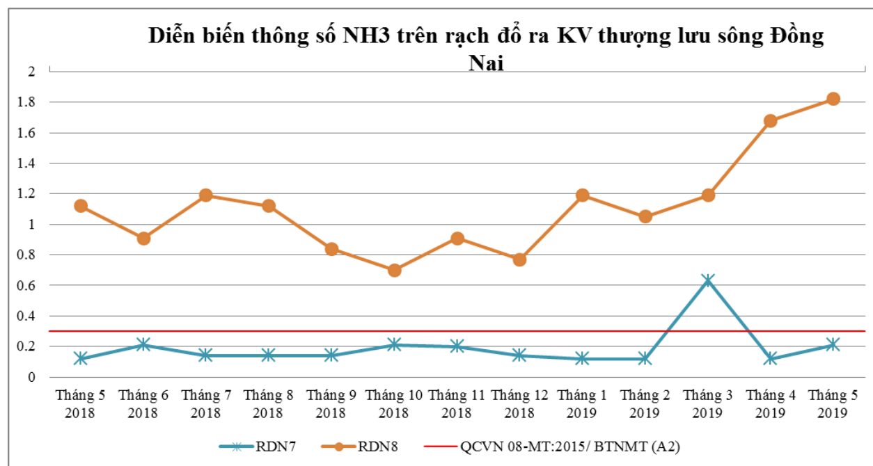
Biểu đồ 11: Diễn biến NH 3 -N trên các rạch đổ ra khu vực thượng lưu sông Đồng Nai
