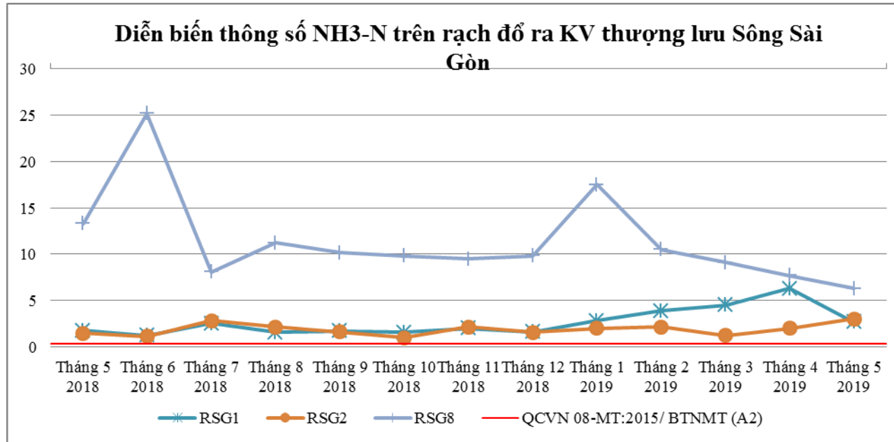
Biểu đồ 3: Diễn biến NH 3 -N trên các rạch đổ ra khu vực thượng lưu sông Sài Gòn
