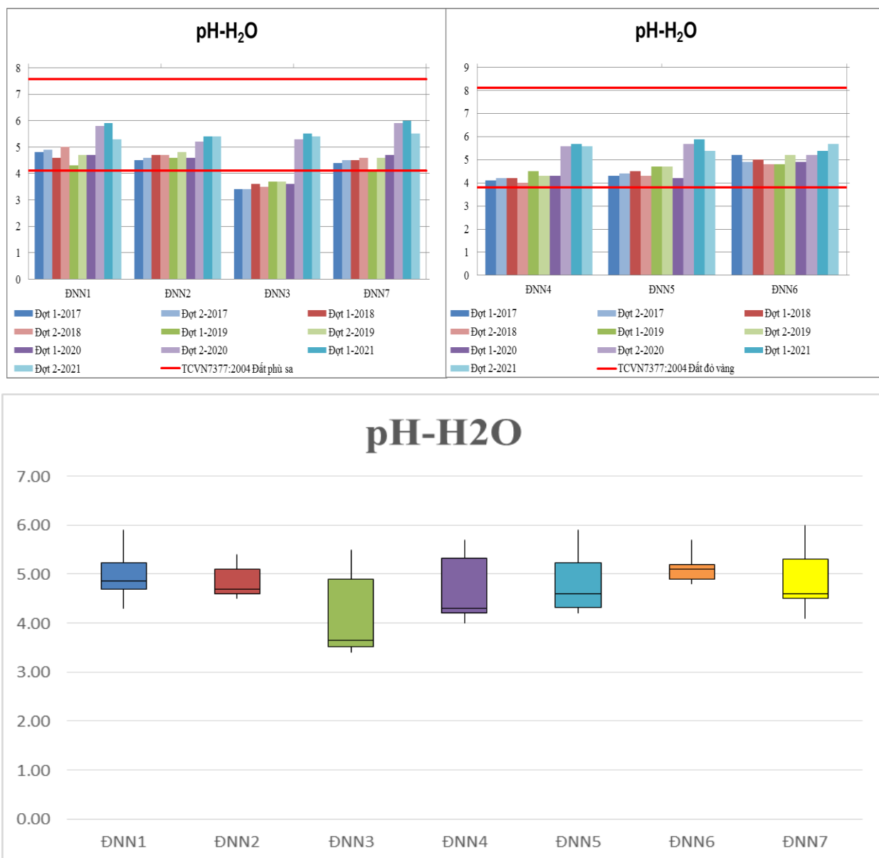
Biểu đồ 7: Giá trị pH H2O tại một số vị trí quan trắc đất nông nghiệp
