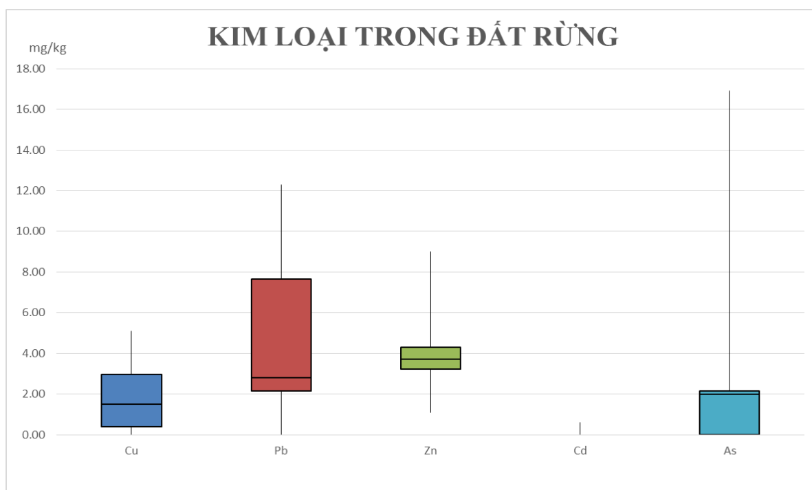
Biểu đồ 17: Hàm lượng kim loại nặng trong đất rừng
