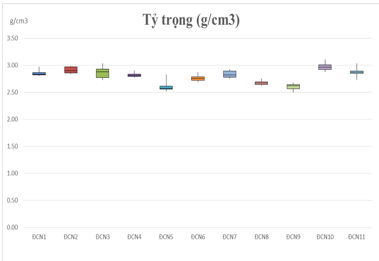
Biểu đồ 4: Tỷ trọng tại các vị trí quan trắc đất công nghiệp
