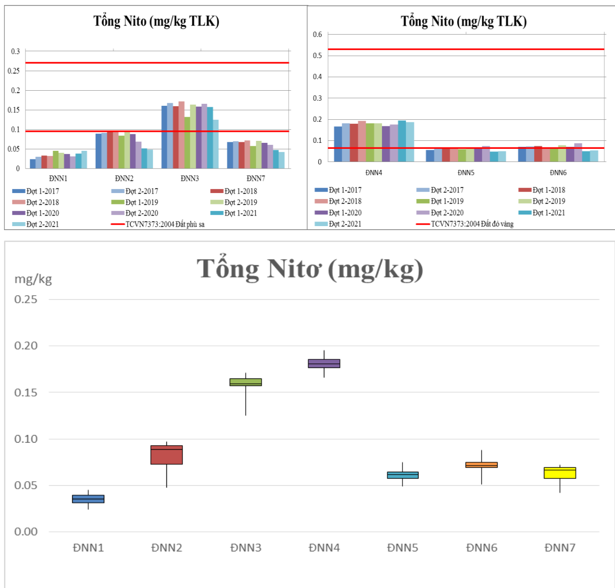
Biểu đồ 12: Hàm lượng nito tổng tại các vị trí quan trắc đất nông nghiệp
