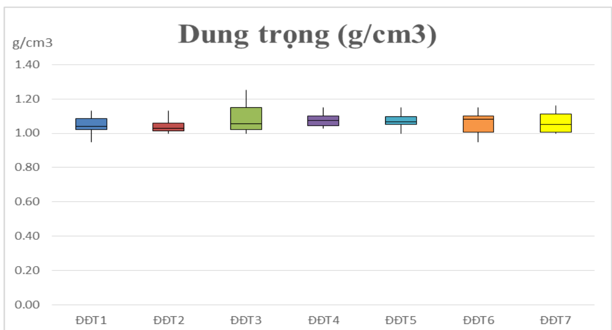
Biểu đồ 19: Dung trọng tại các vị trí quan trắc đất đô thị
