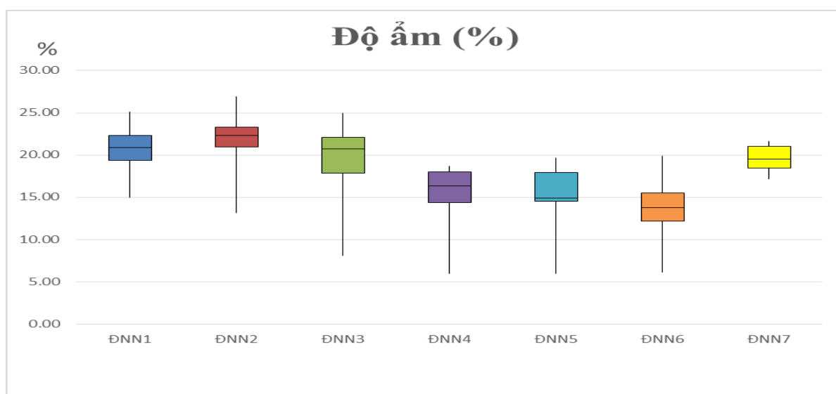
Biểu đồ 9: Độ ẩm tại một số vị trí quan trắc đất nông nghiệp
