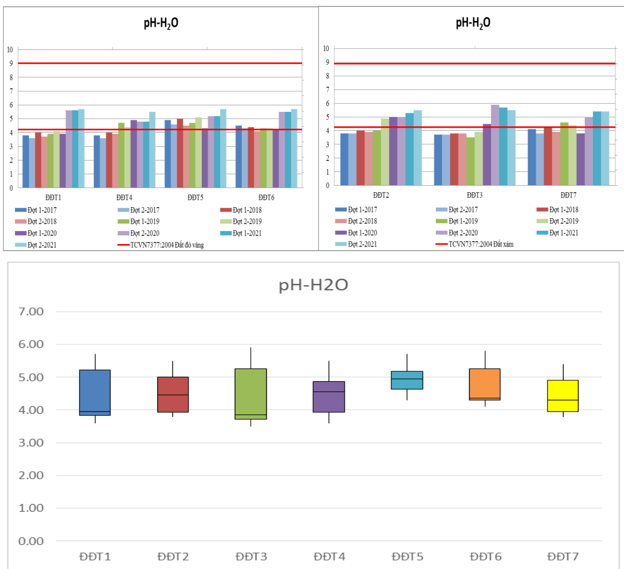
Biểu đồ 15: Giá trị pH H2O tại một số vị trí quan trắc đất đô thị
