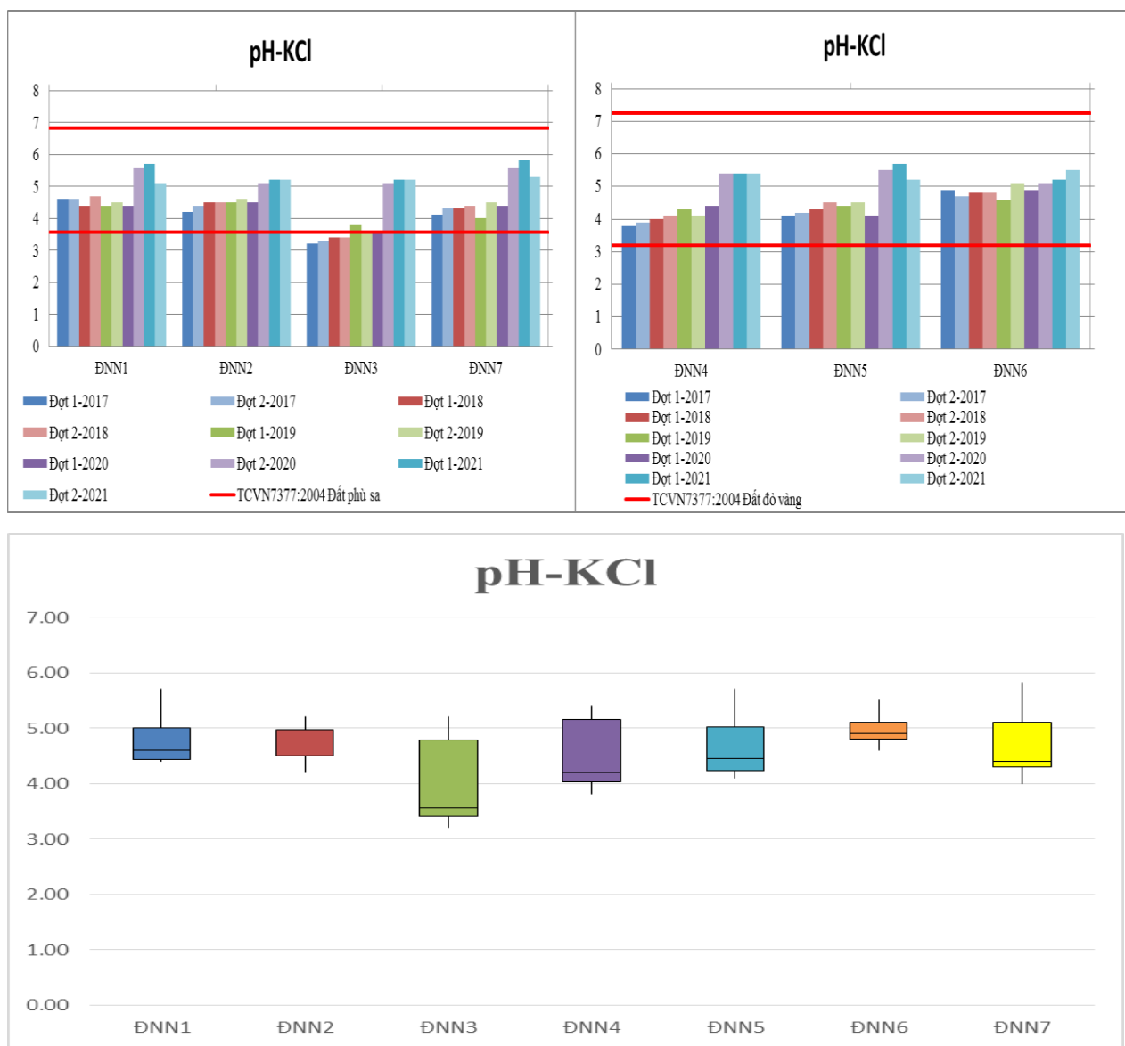
Biểu đồ 8: Giá trị pH_{KCl} tại các vị trí quan trắc đất nông nghiệp
