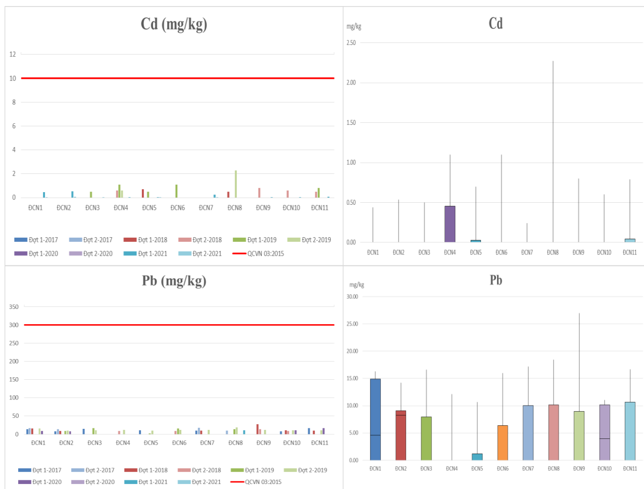
Biểu đồ 6: Hàm lượng kim loại nặng đất công nghiệp
