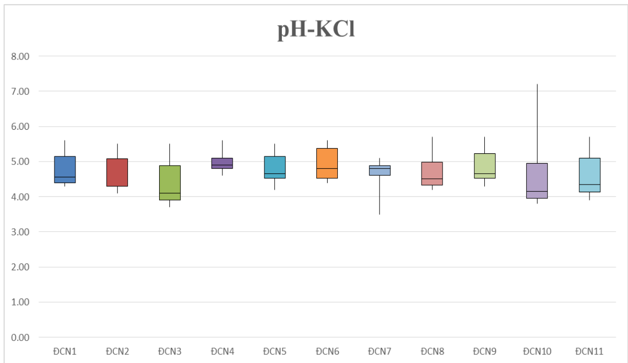
Biểu đồ 2: Giá trị pH KCl tại các vị trí quan trắc đất công nghiệp
