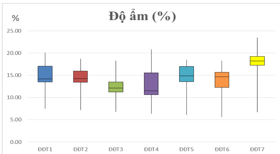
Biểu đồ 107: Độ ẩm tại một số vị trí quan trắc đất đô thị
