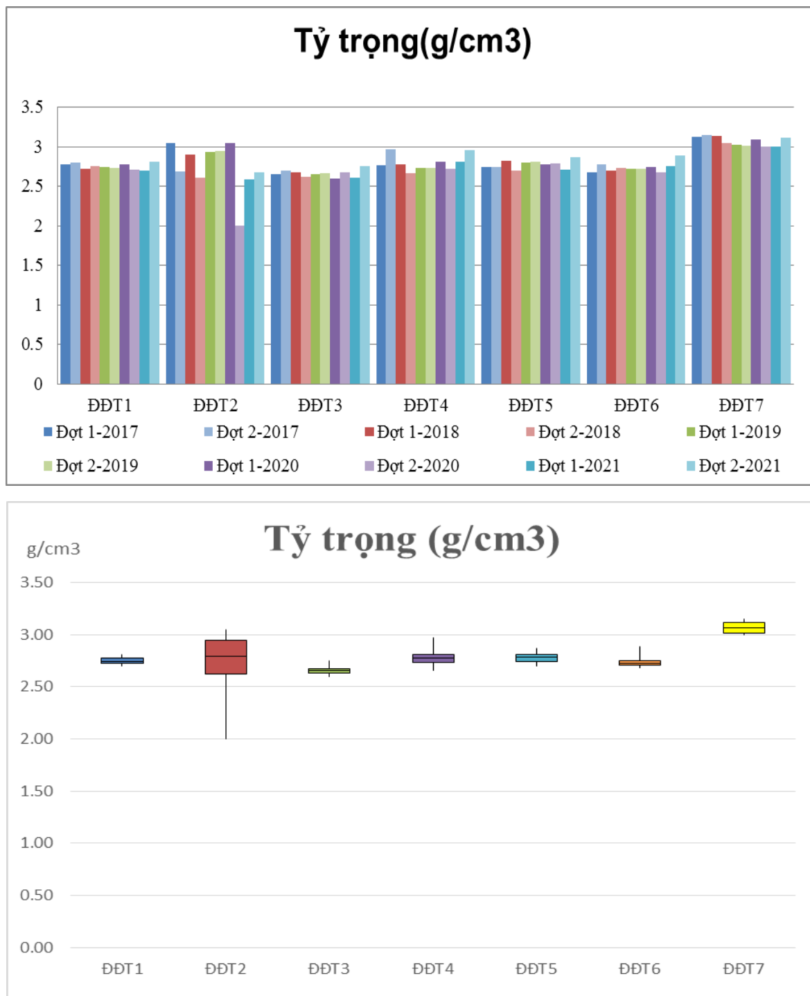
Biểu đồ 118: Tỷ trọng tại các vị trí quan trắc đất đô thị.
