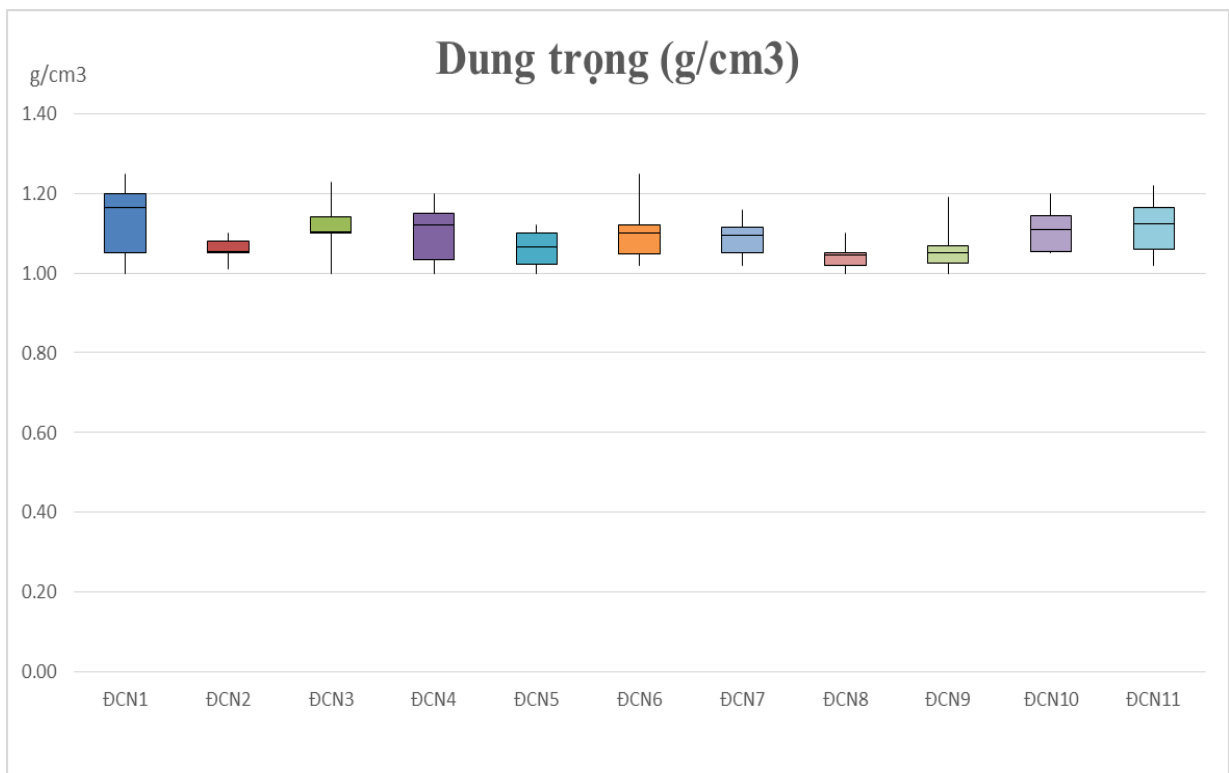
Biểu đồ 5: Dung trọng tại các vị trí quan trắc đất công nghiệp
